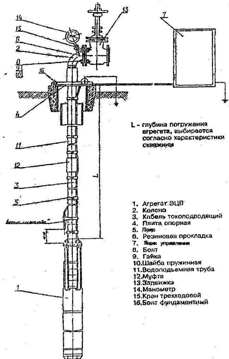
Рис. 1 Расположение агрегата в скважине
