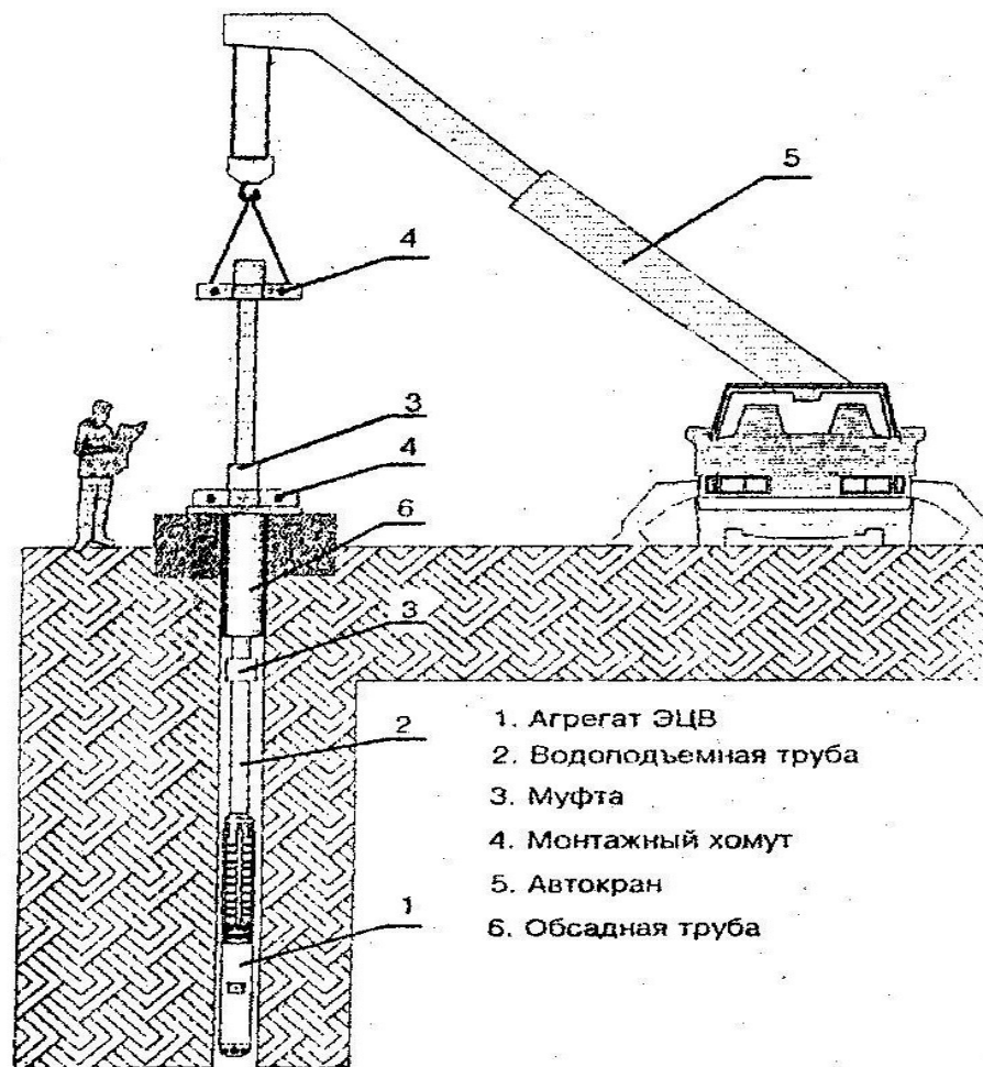
Рис.3 Монтаж агрегата в скважину
